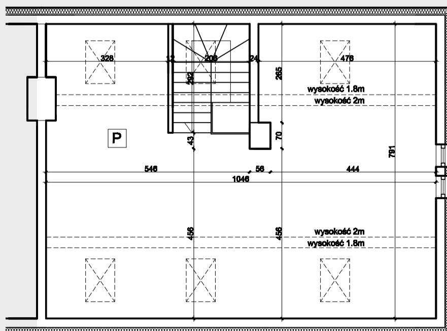
PODDASZE
